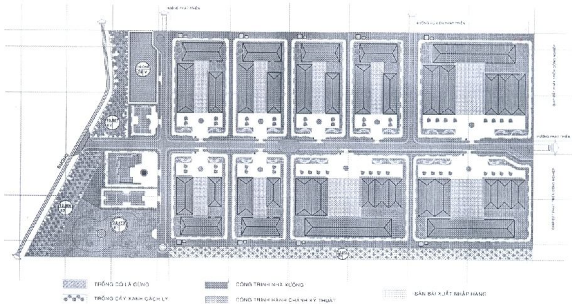
Sơ đồ quy hoạch xây dựng cụm công nghiệp- tiểu thủ công nghiệp tại xã Thăng Hải, huyện Hàm Tân, tỉnh Bình Thuận
