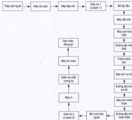
Hình 4: Quy trình sản xuất tôn mạ màu liên tục
