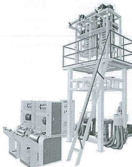
Máy thổi đơn lớp 2 đầu hình
